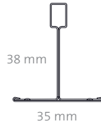
Primario 3600 mm
