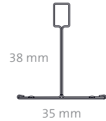
Secundario 600 mm
